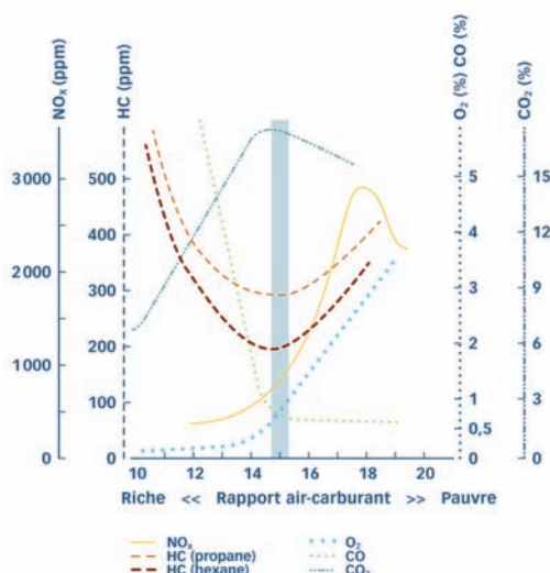
Figure 2 : Équilibre des gaz de combustion pour un rapport idéel air- carburant (propane)
